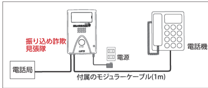
図2 機械配線図
