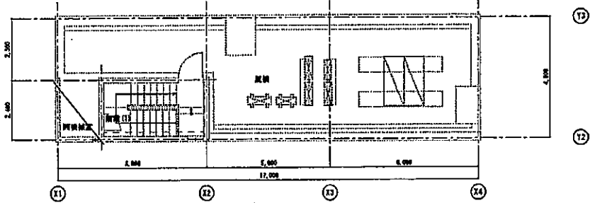
PH階平面図 1/100
