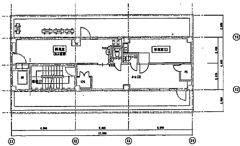
4階平面図 1/100
