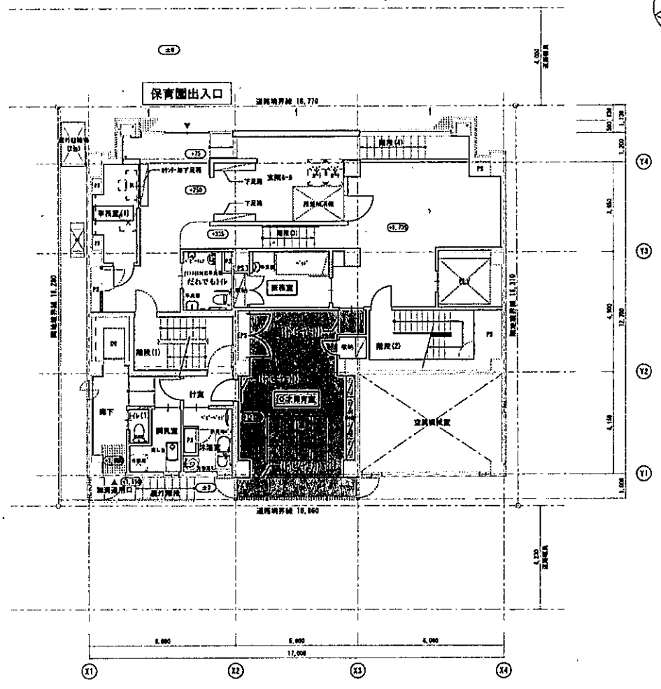
1階平面図 1/100
