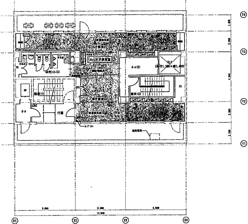
3階平面図 1/100
