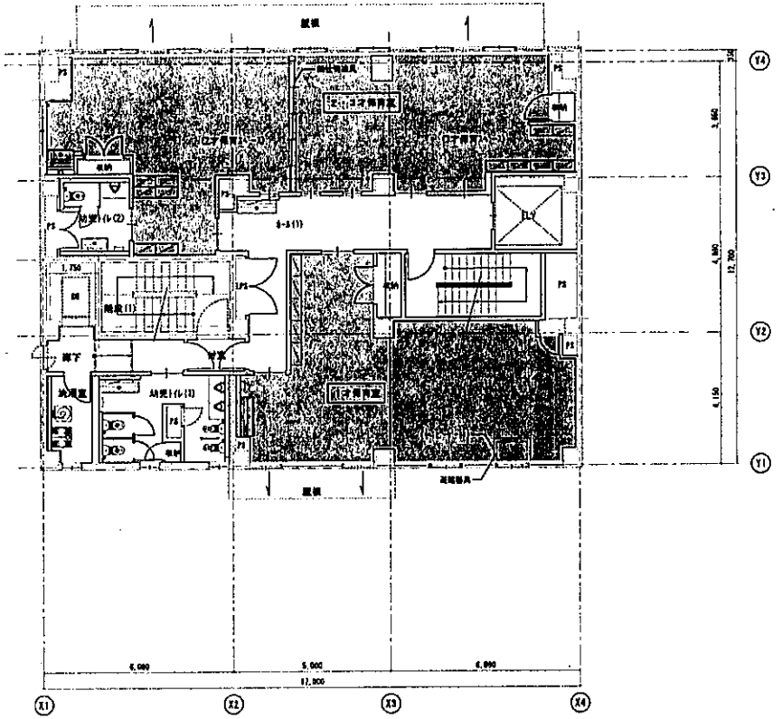
2階平面図 1/100
