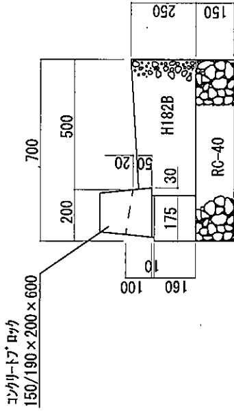
街渠詳細図
