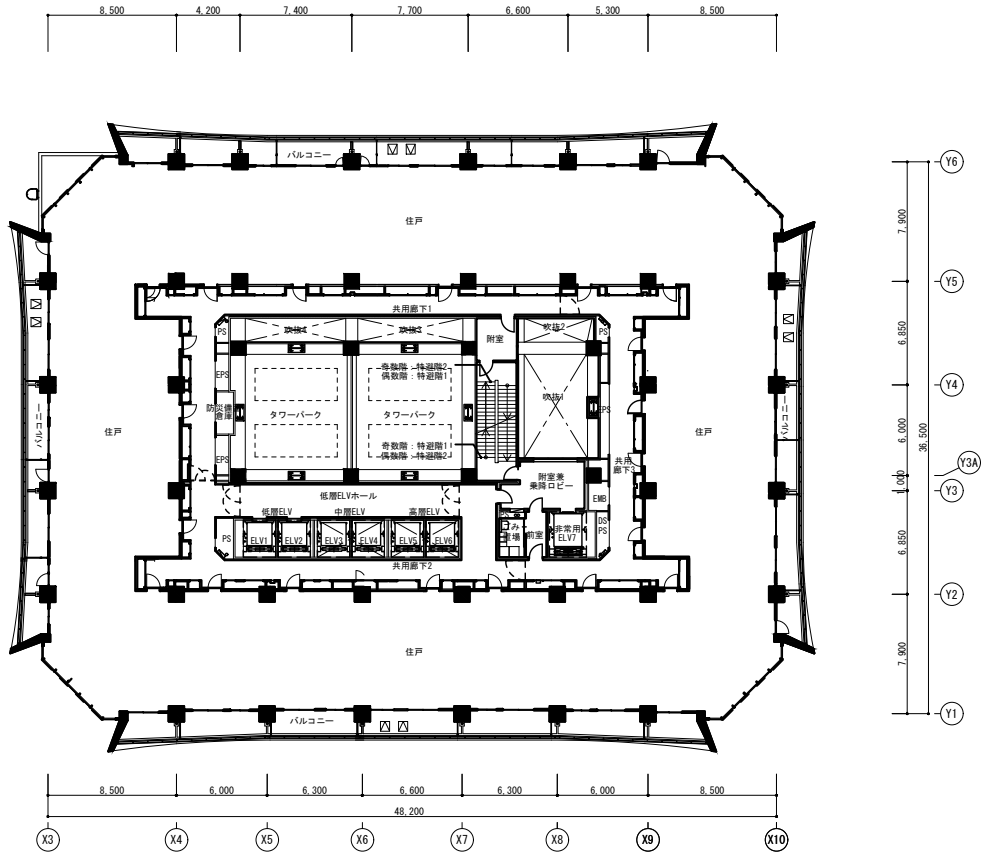
5階平面図
