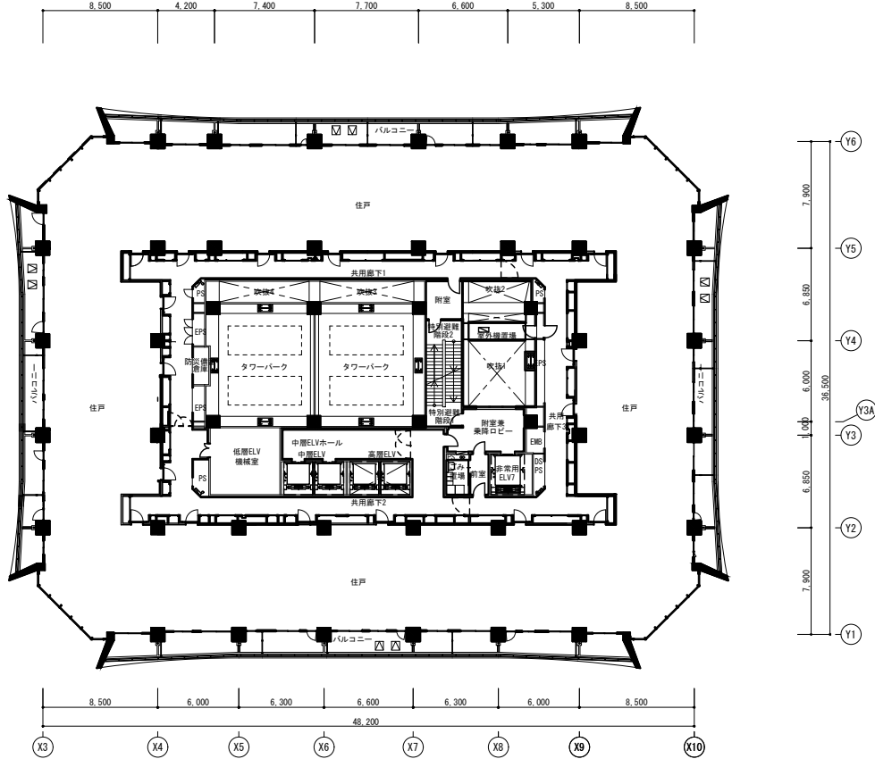
21階平面図
