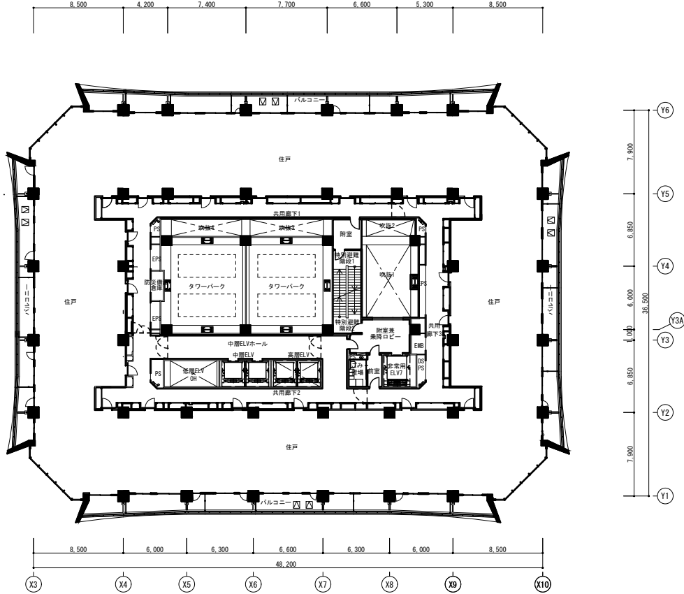
20階平面図
