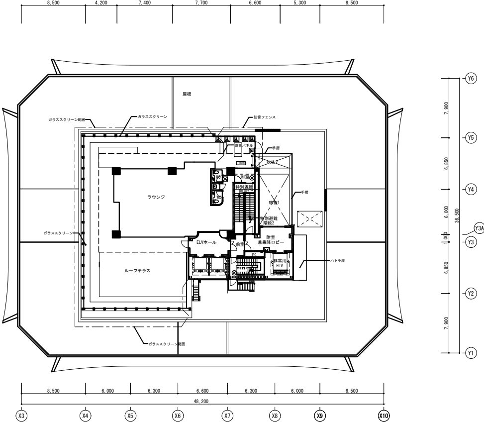
PH階平面図
