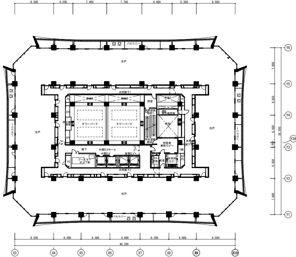
22階平面図
