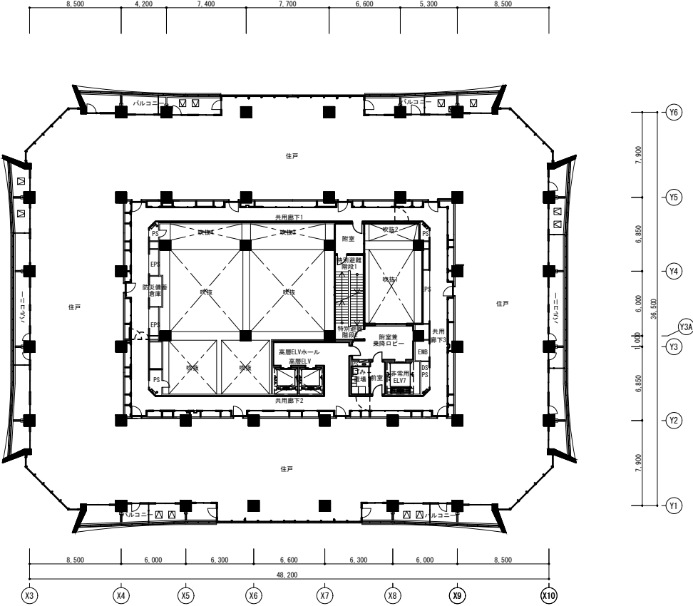
46階平面図
