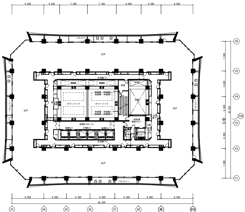
6～7階平面図
