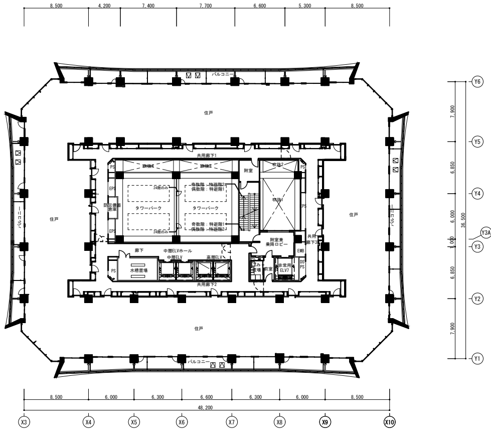
25～30階平面図
