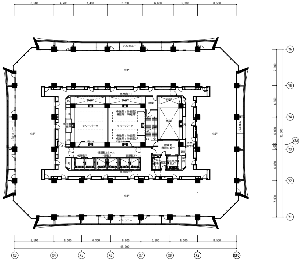
8～13階平面図
