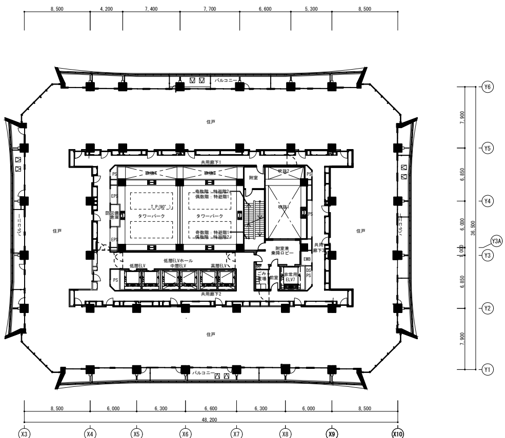
14～19階平面図
