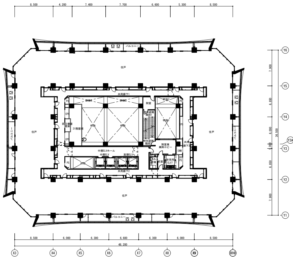
32階平面図
