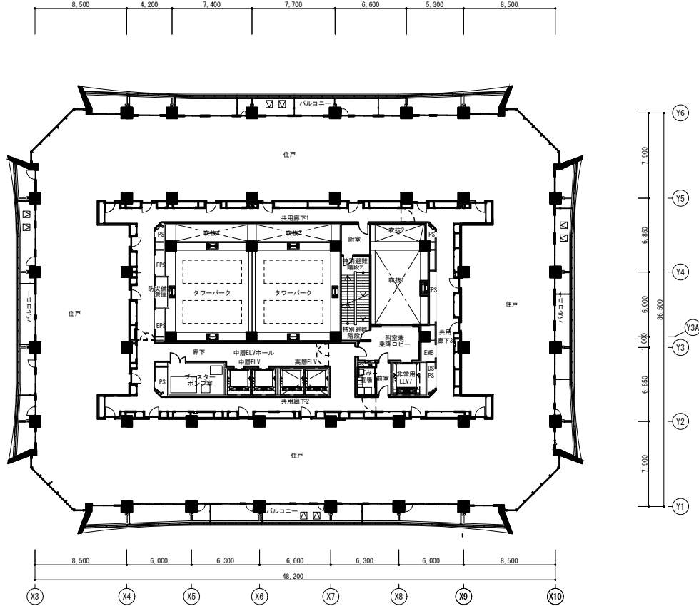
23階平面図
