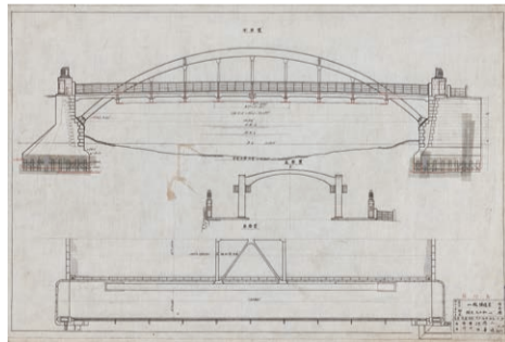
▲ 震災復興橋梁図面(稲荷橋)
