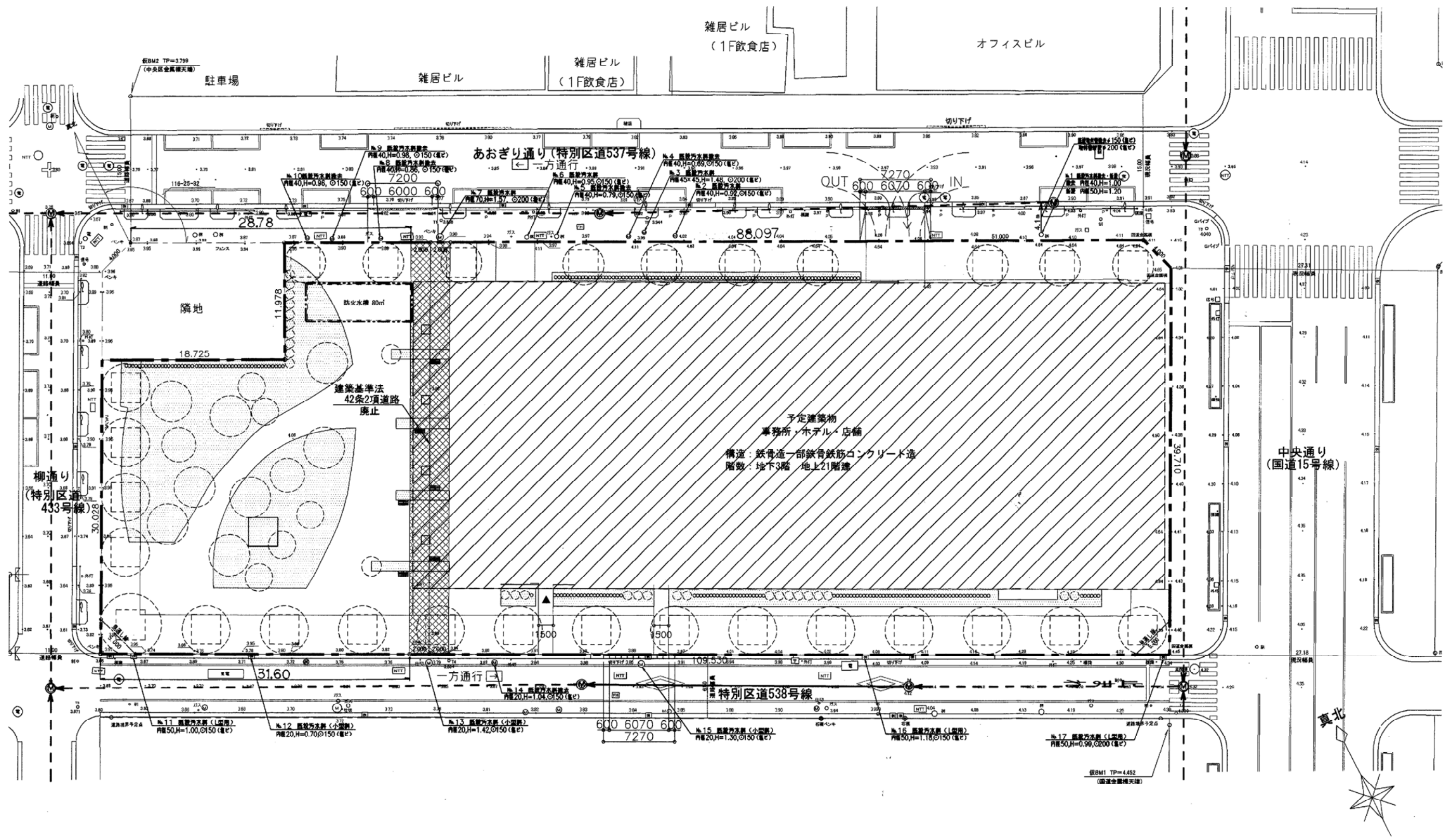
土地利用計画図 1/400
