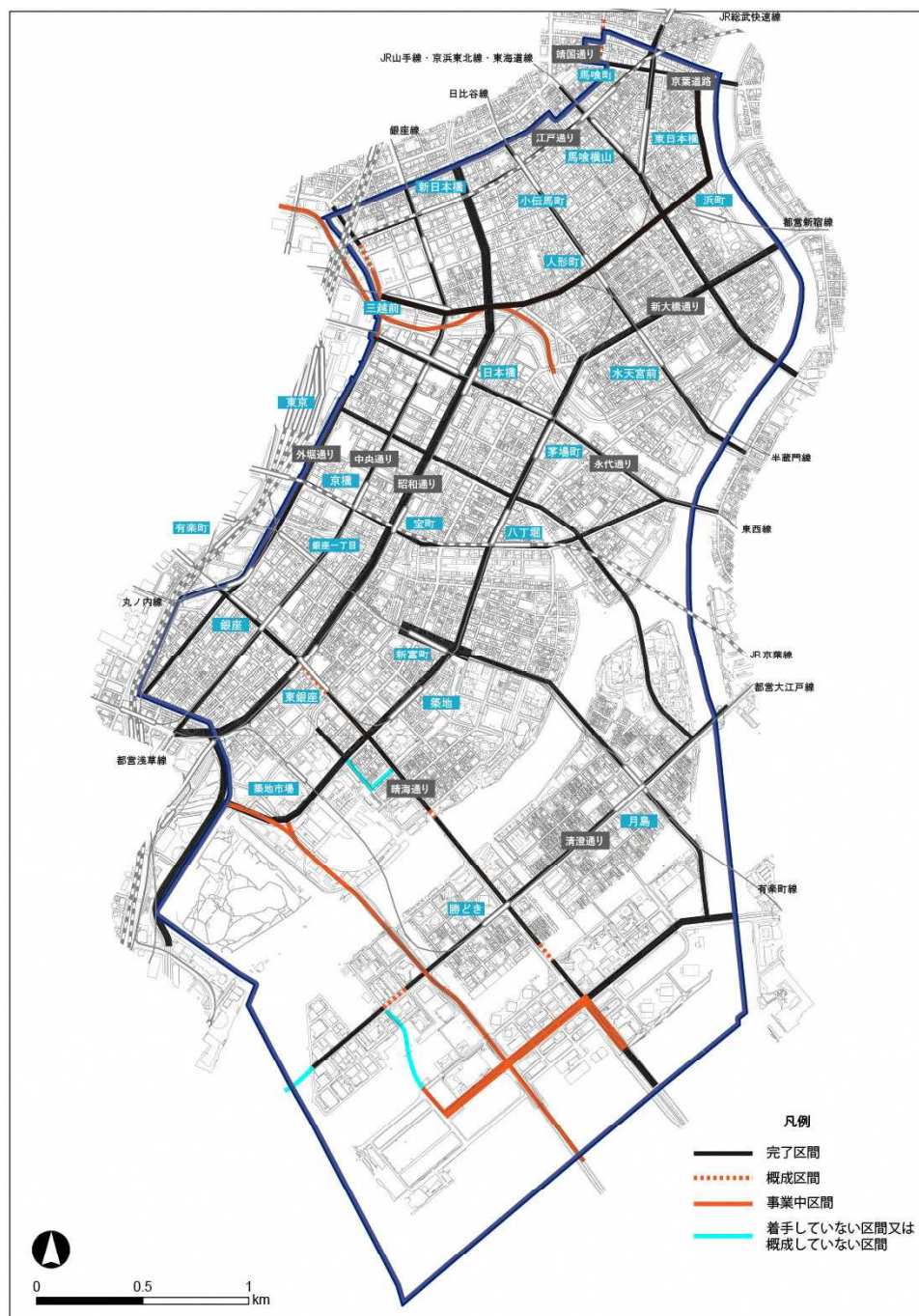
図 31 都市計画道路線網図
