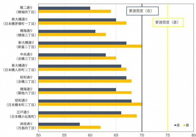
図 36 自動車騒音
