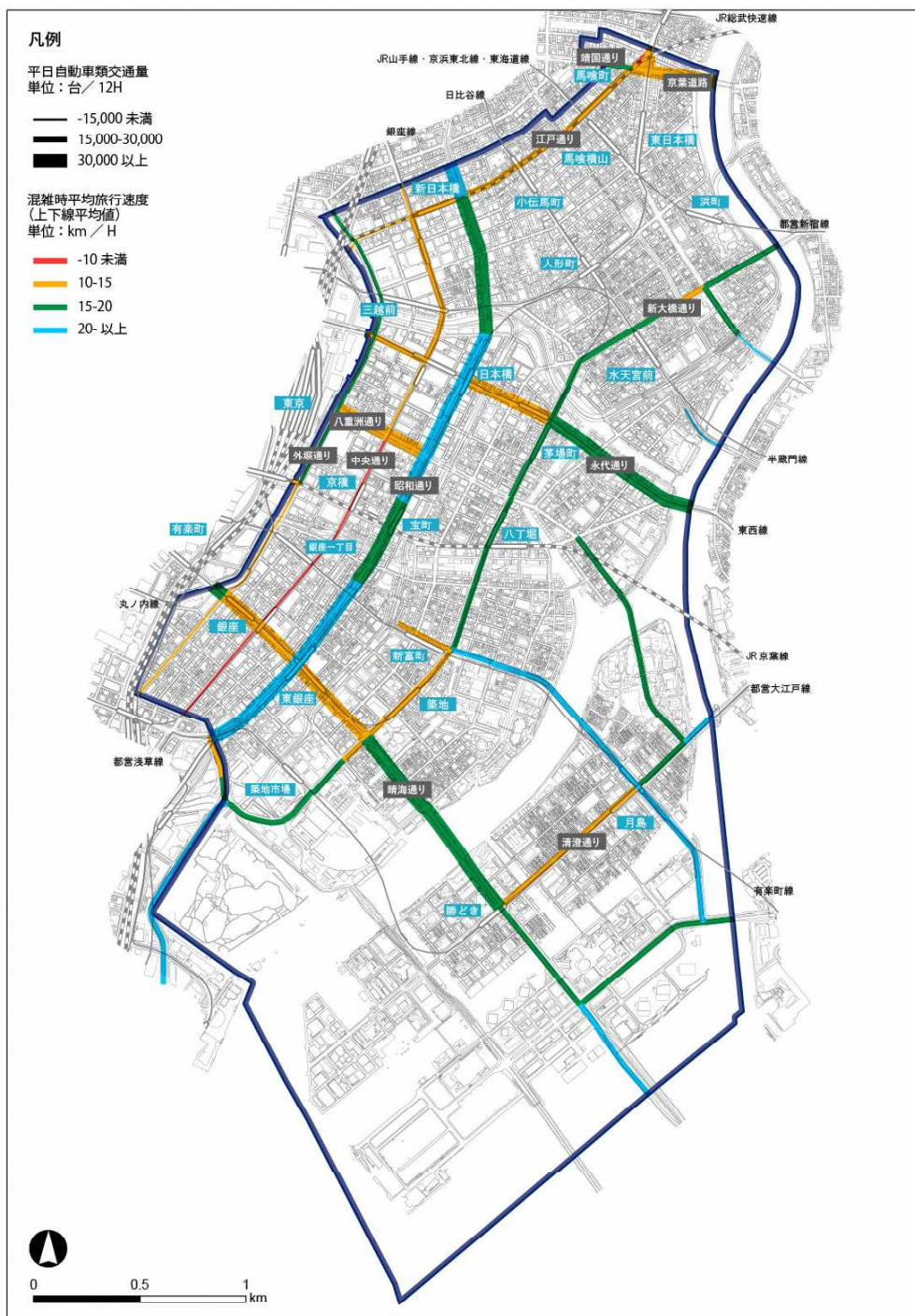
図 32 区内道路（一般道）の交通量と混雑時平均旅行速度
