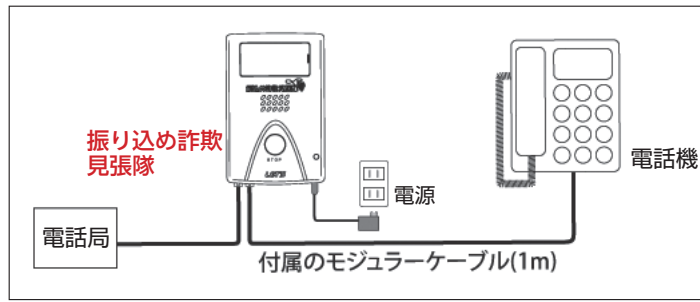
図2 機械配線図
