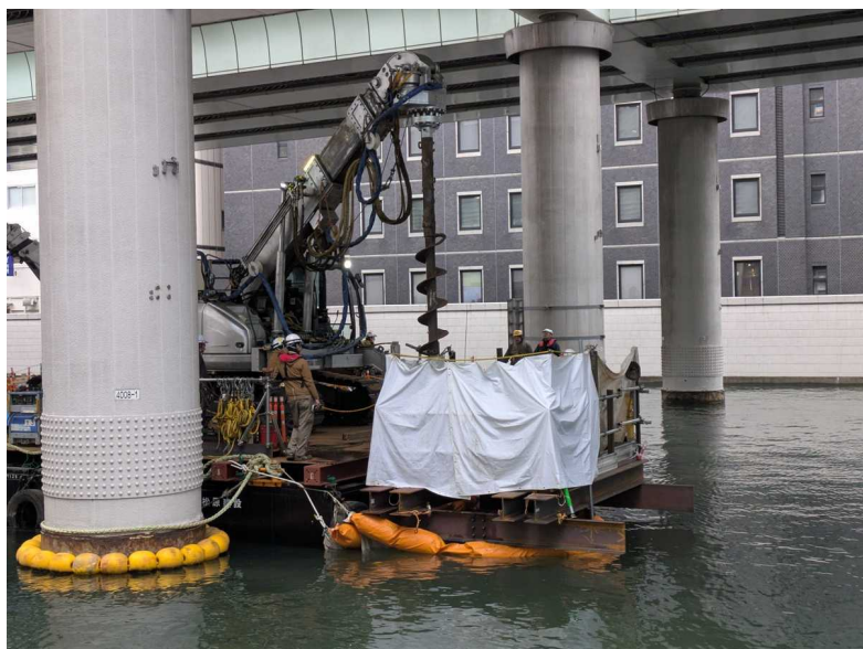
写真1 準備工事状況（仮受橋脚・日本橋上流側）
