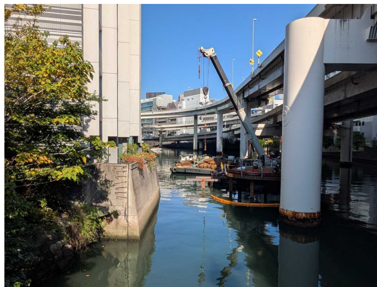
写真2 準備工事状況（う回路橋脚・鰐橋上流側）
