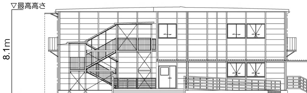
東面 立面図
