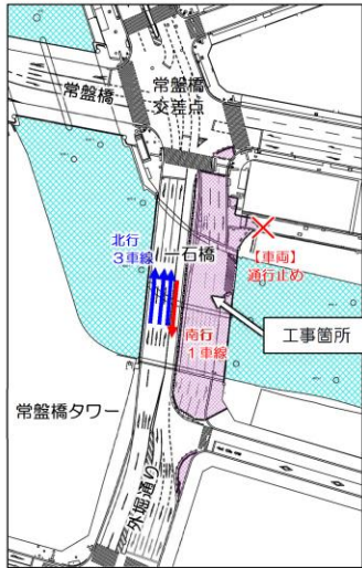
切回し後の車線形状
