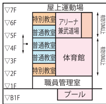
各階諸室配置案
