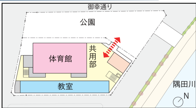
平面諸室配置案
