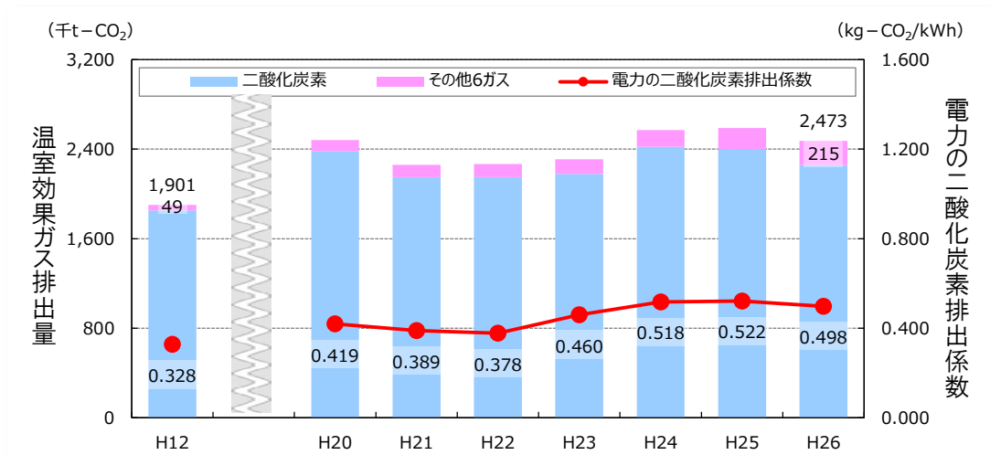
図2-9 これまでの中央区の温室効果ガス排出量
