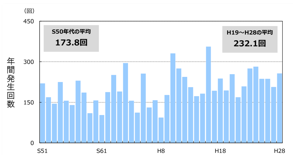
図 2-20 1時間降水量 50mm 以上の年間発生回数(1,000 地点当たり)
