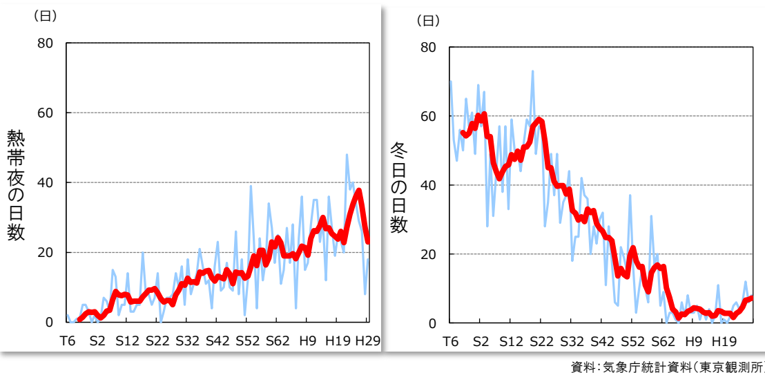
図2-18 東京における熱帯夜※(左)と冬日※(右)の日数の推移(過去100年)
